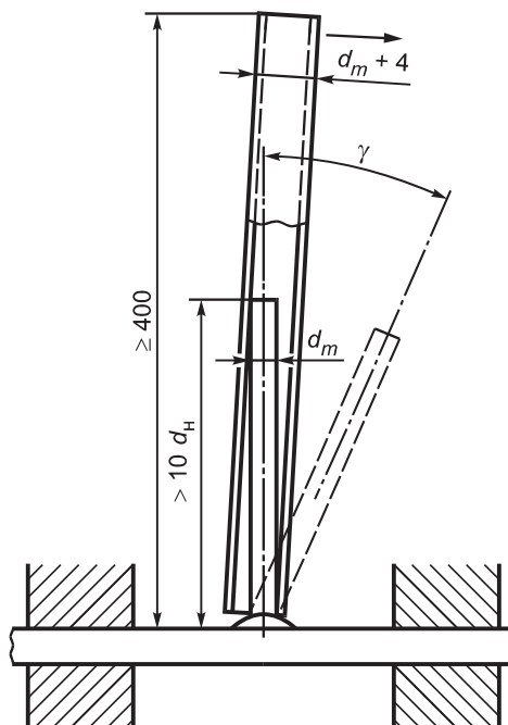
d_H — номинальный диаметр рабочей арматуры; d_m — максимальный размер поперечного сечения испытуемого арматурного проката
