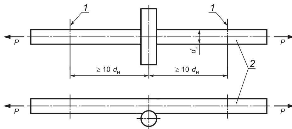
P — испытательная нагрузка; 1 — граница закрепления в захватах разрывной машины; 2 — стержень рабочей арматуры; d_H — номинальный диаметр рабочей арматуры
