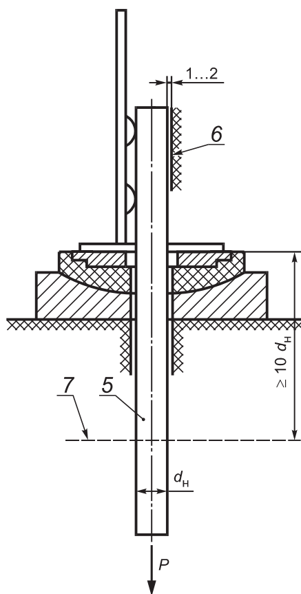
Рисунок 4 — Схема испытания нахлесточных соединений анкерных стержней закладных изделий на срез
