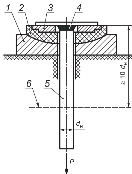
Рисунок 3 — Схема испытания тавровых соединений анкерных стержней закладных изделий на отрыв
